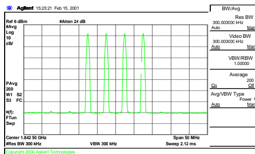
Fig. 5. GSM output spectrum
